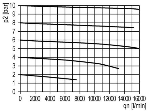
Durchflussdiagramm
